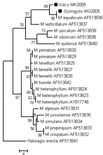
2. ábra „Legnagyobb takarékoság” eljárással készült konszenzus törzsfá a két új hazai süllőhínár minta (Kácsi-patak: Kács, Tarnóca-patak: Gyöngyös) és más süllőhínár fajok ITS szekvenciáinak bevonásával. A fa szerkesztése, 1000 véletlenszerű ismétlést (bootstrap) figyelembe véve, a MEGA 3.1 programcsomag „Maximum Parsimony” algoritmusának felhasználásával történt. A törzsfát Haloragis erecta ITS szekvenciájával gyökerezítettük. A skála a nukleotidcserék számát jelöli. A törzsfán szereplő süllőhínár ITS-szekvenciák az EMBL adatbázisból származnak az ottani azonosító kódjaikkal:
